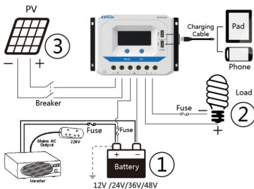
Obrázek 2 Schéma zapojení
